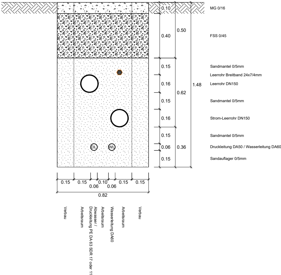
Leitungsgraben RQ ungebunden:
