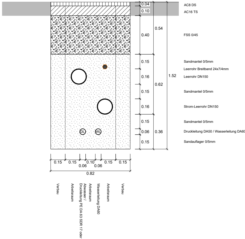
Leitungsgraben RQ gebunden:
